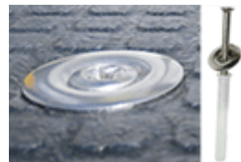
KRAIBURG upínací systém: mimoriadne robustné, zaoblené a zapustené s podložkou
